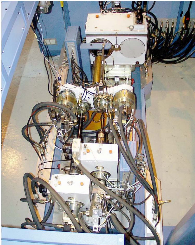
Die Abbildung zeigt die Antriebs- und Belastungseinheit mit aufgespanntem Prüfling AMAD (P/N 42312-26) F/A-18.
