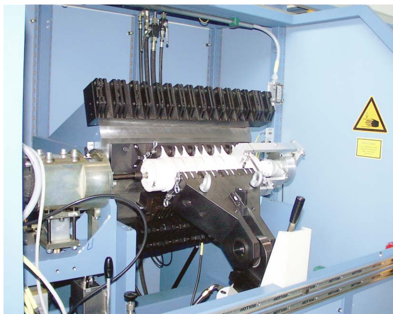
Die Abbildung zeigt die Transmission-Einheit mit aufgespanntem Prüfling LEADING EDGE FLAP RH (P/N 2022636-4-4) F/A-18.
